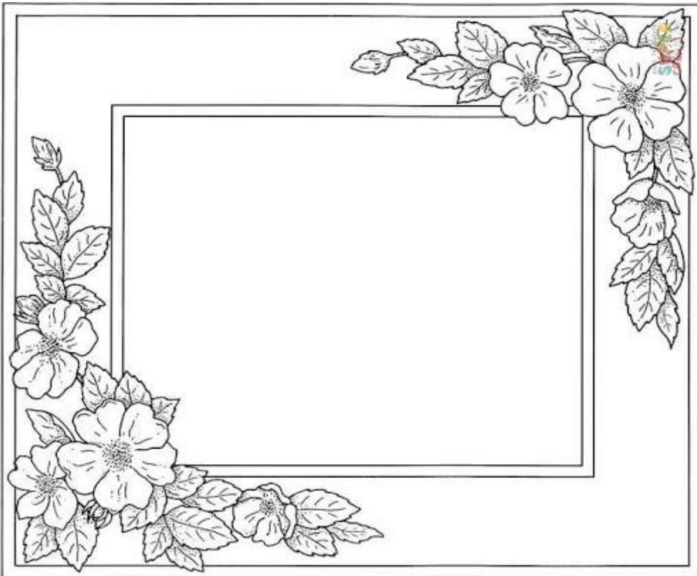
Ilustración 3. Marcos Google
